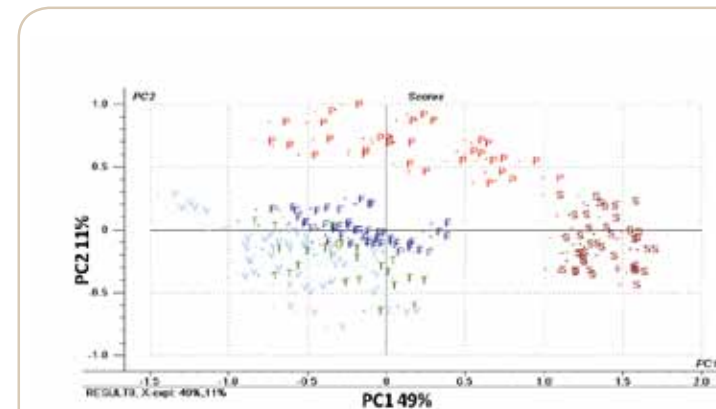
Figure 2 Analyse en composante principale des spectres infrarouge des parois de tige de blé après action de cellulases.
