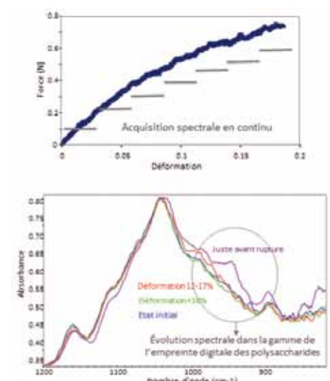
Figure 3 Test de traction sur une éprouvette de couche à aleurone ablatée et soniquée. Courbe force/déformation et spectres IR acquis pour différentes phases de déformation.
