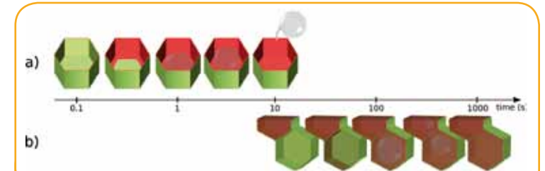
Figure 3 Interprétation de la percolation biphasique huile (en rouge)/air (en gris) à l'échelle cellulaire : a) cellule tronquée en contact avec un film d'huile ; b) migration de l'huile entre les couches 1 et 2.
