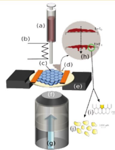
Figure 1 Configuration du dispositif sur la platine du microscope TELEMOS. (a) micro-seringue permettant de déposer un volume d'huile contrôlé ; (b) aiguille chauffée ; (c) échantillon équilibré au préalable avec de la vapeur d'eau surchauffée ; (d) surplaque chauffée ; (e) objectif (x10 ou x40) ; (f) objectif (x10 ou x40) ; (g) rayonnement synchrotron ; (h) percolation dans le plan vertical ; (i) parenchyme de pomme de terre (vitreux dans les conditions de mesure) ; ou (j) enrobage avec panure (idem).
