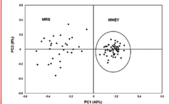
Figure 2 Représentation graphique de la variation de la dérivée seconde des spectres obtenus dans la région 2870 – 2840 \text{cm}^{-1} (bande d'élongation symétrique des groupements \text{CH}_2 correspondant aux lipides de membrane). Les cellules cultivées dans du MRS ont montré une grande hétérogénéité dans le comportement lipidique, tandis que les cellules cultivées dans du lactosérum doux ont présenté un comportement de cluster plus homogène.
