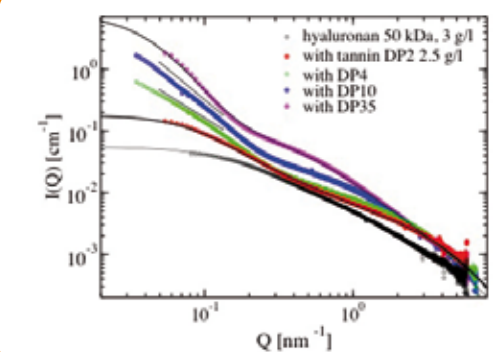
Figure 3 Effet du degré de polymérisation des tanins sur les profils SAXS du système tanin-polysaccharide.
