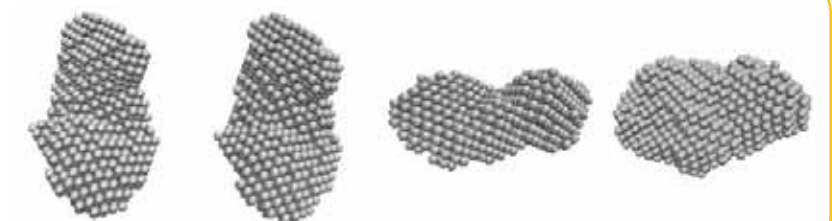
Figure 3 Modèle 3D basse résolution le plus probable d'un oligomère de AtPP2-A1.
