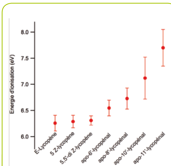
Figure 2 Énergie d'ionisation du E -lycopène, de ses isomères Z et de ses produits d'oxydation.
