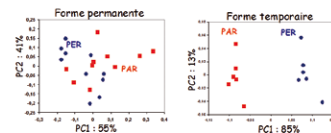
Figure 2 Discrimination des spectres PER et PAR obtenus sur des échantillons sous la forme permanente et temporaire.
