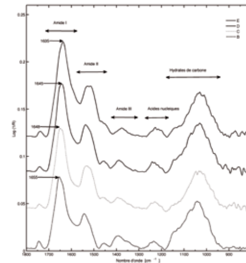
Figure 2 Spectres FTIR bruts des levures S. cerevisiae et régions spectrales caractéristiques (1800 – 800 cm -1 ), pour les échantillons suivants : (B) levures "fraîches", cultivées en milieu YPD gélosé puis resuspendues dans de l'eau déionisée ; (C) levures après 24 h en suspension dans une solution saline (NaCl 0,15 M) ; (D) levures après 24 h de contact avec la matrice organosiliciée en solution saline ; (E) levures après 24 h de contact avec le revêtement nanocomposite en solution saline. La position du pic amide I est indiquée sur la figure. À noter que, par souci de clarté, ne figurent pas les données relatives aux levures après 2 h d'exposition à l'argent ionique (AgNO 3 2 mM dans eau déionisée).
