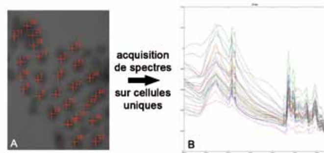
Figure 1 Spectres FTIR sur cellules uniques de S. cerevisiae exprimant AtClo1 après 42 heures de culture. A , image en lumière visible de cellules séchées sur hémisphère de ZnSe. B , spectres obtenus à partir de cellules d'un même hémisphère.
