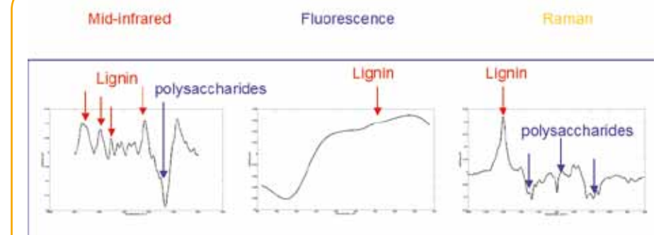
Figure 2 Profils spectraux obtenus par analyse de co-inertie : composante 2.
