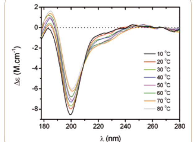
Figure 2 Spectres SRCD d'une sous-unité gluténine de haut poids moléculaire (HMW-SU) en 20 mM NaF pH 7.2 en fonction de la température.
