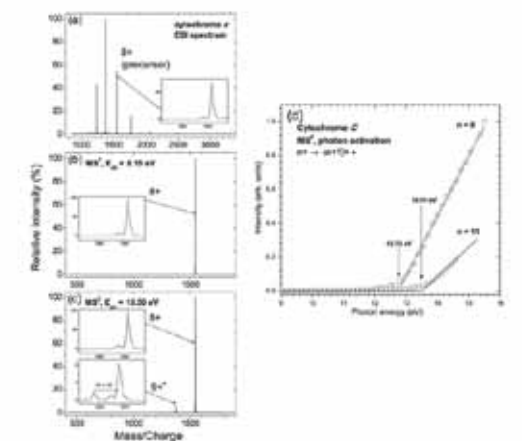
Figure 3 (a) Spectre ESI d'une solution aqueuse de cytochrome C montrant l'ion précurseur. (b) Spectre de masse consécutif à l'irradiation du précurseur à 8.15 eV pendant 80 ms. (c) Spectre de masse consécutif à l'irradiation du précurseur durant 80 ms à 15.5 eV. (d) Rendements de photoionisation enregistrés pour deux pré-curseurs entre 9 et 15.5 eV. L'ajustement aux données expérimentales d'une loi de seuil (lignes continues) permet l'obtention des seuils d'ionisation.
