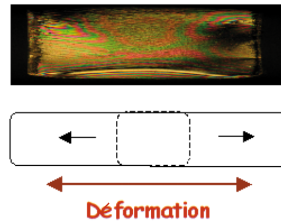
Figure 1 Visualisation des contraintes résiduelles en lumière polarisée au sein d'un échantillon amorphe vitreux sous forme temporaire.
