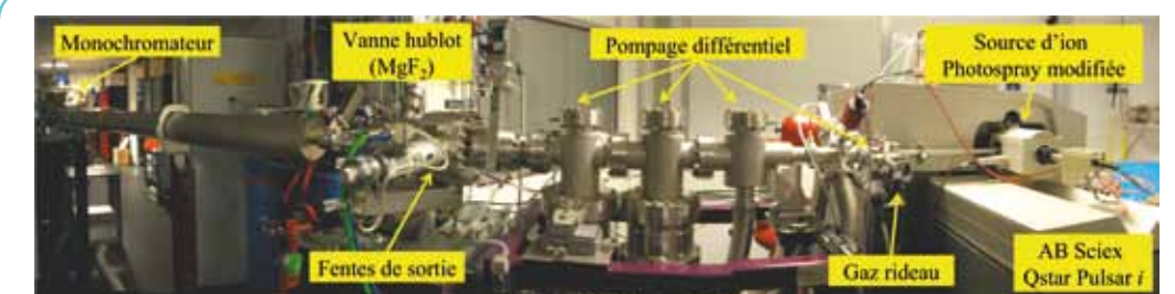
Figure 3 Photographie panoramique de la branche APEX avec le dispositif de photoionisation à pression atmosphérique.
