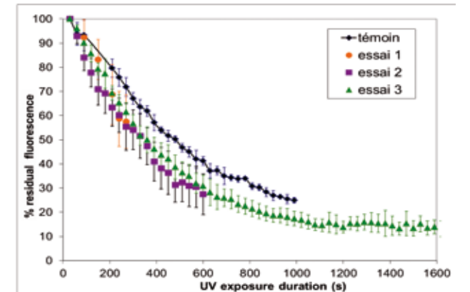
Figure 3 Perte de fluorescence du \beta -carotène en fonction de la durée d'exposition au rayonnement UV de l'émulsion témoin sans induction et de trois émulsions avec induction de l'oxydation par le réactif de Fenton.
