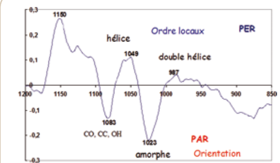
Figure 3 Tracé du premier vecteur propre de l'ACP sur les spectres IR de la forme temporaire révélant les bandes associées aux structures parallèles et perpendiculaires au plan de polarisation du faisceau infrarouge.
