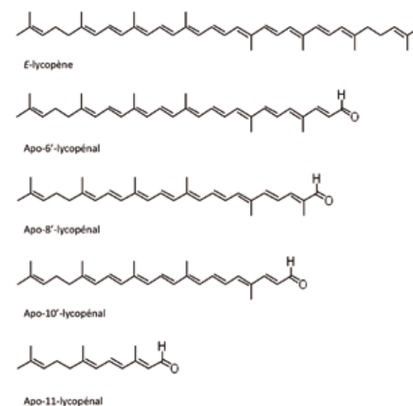
Figure 1 Structure chimique du E -lycopène et de ses produits d'oxydation étudiés.
