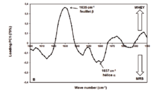
Figure 1 (A) Représentation graphique de la variation de la dérivée seconde des spectres dans la région amide I (1700 – 1600 \text{cm}^{-1} ) en fonction du milieu de culture, dans le plan 1-2 de l'ACP. La composante 1 (PC1) permet de différencier les cellules sur la base du milieu de culture. (B) Les cellules cultivées dans du lactosérum présentent un décalage significatif du pic ( \sim 30 \text{ cm}^{-1} ) (i.e. plus des structures secondaires en feuillet \beta en comparaison aux cellules cultivées dans du milieu MRS (i.e. plus de structures secondaires hélice \alpha ).
