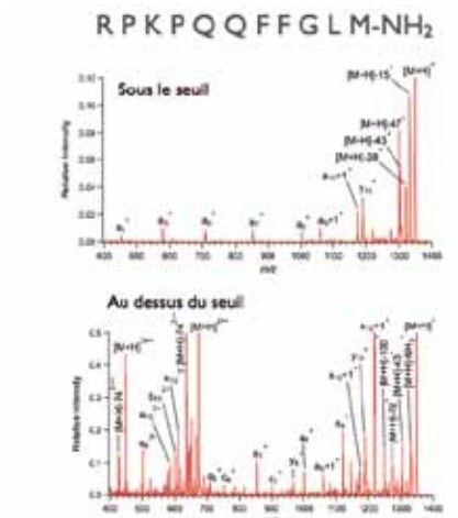
Figure 2 Spectre de masse tandem pour la substance P après irradiation à 8 eV (sous le seuil d'ionisation) et à 15 eV (au-dessus du seuil d'ionisation).
