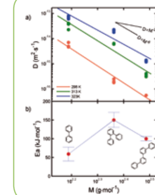
Figure 2 a) Coefficient de diffusion d'oligophényles ( n=2,3,4 ) dans un polypropylène (cristallinité = 30 %) et b) énergie d'activation correspondante.
