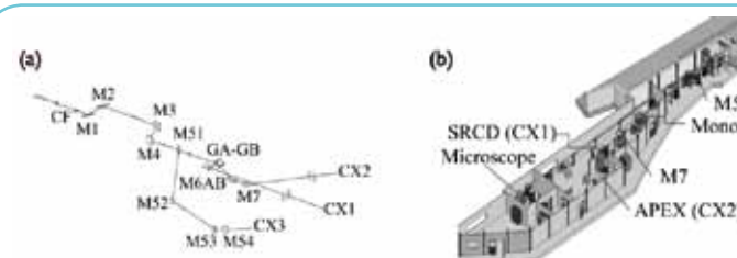
Figure 1 (a) Schéma optique de la ligne DISCO, comprenant les éléments optiques et leur distance à la source. (b) Plan d'installation de la ligne.
